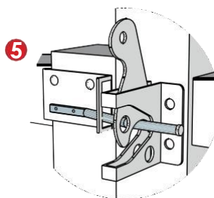
Exemple de loquet installé à l'intérieur de l'enceinte
